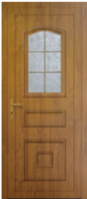
Vega 1L Vitrage feuilleté Croisillons laiton en option U D = 1,5 W/m 2 .K Chêne doré
