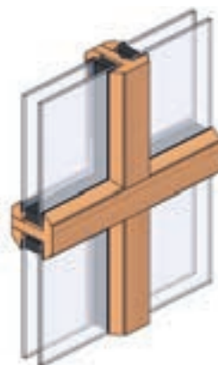
Petits bois mortaisés Petit bois mortaisé largeur 53 mm. Il est assemblé par tenon dans le vantaill. C'est le petit bois traditionnel adapté aux normes actuelles.
