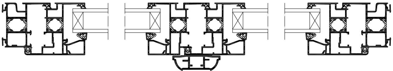
Frappe traditionnelle : design droit intégral
